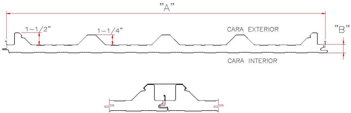
Detalle Unión
